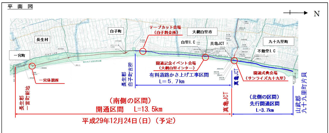
平面図
