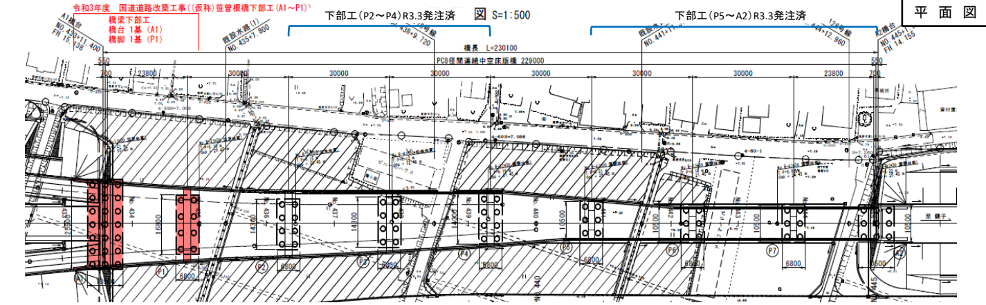
側面図
