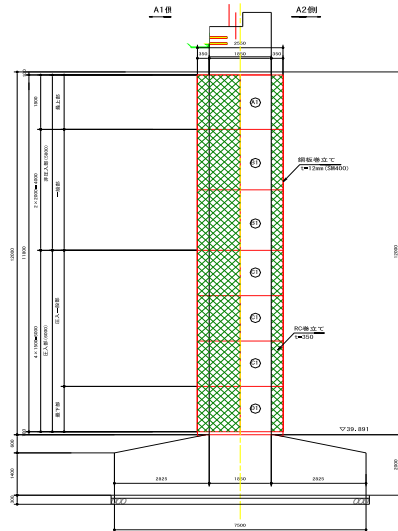
断面図
